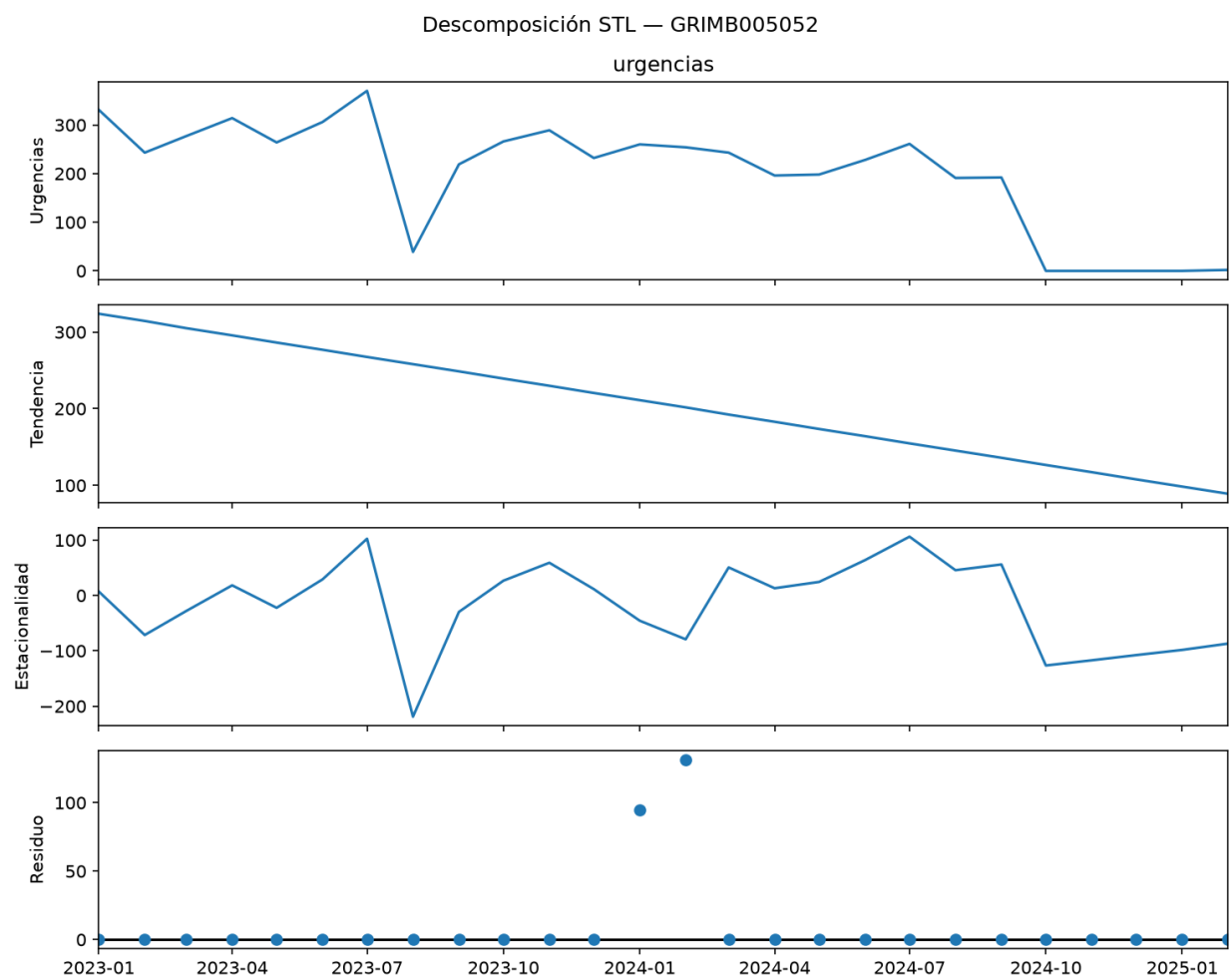
Figura 4: Descomposición STL
