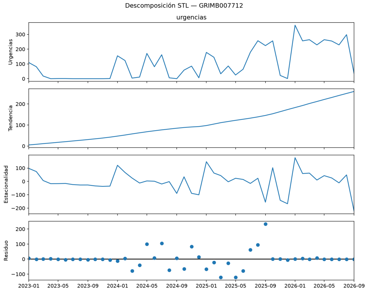
Figura 6: Descomposición STL
