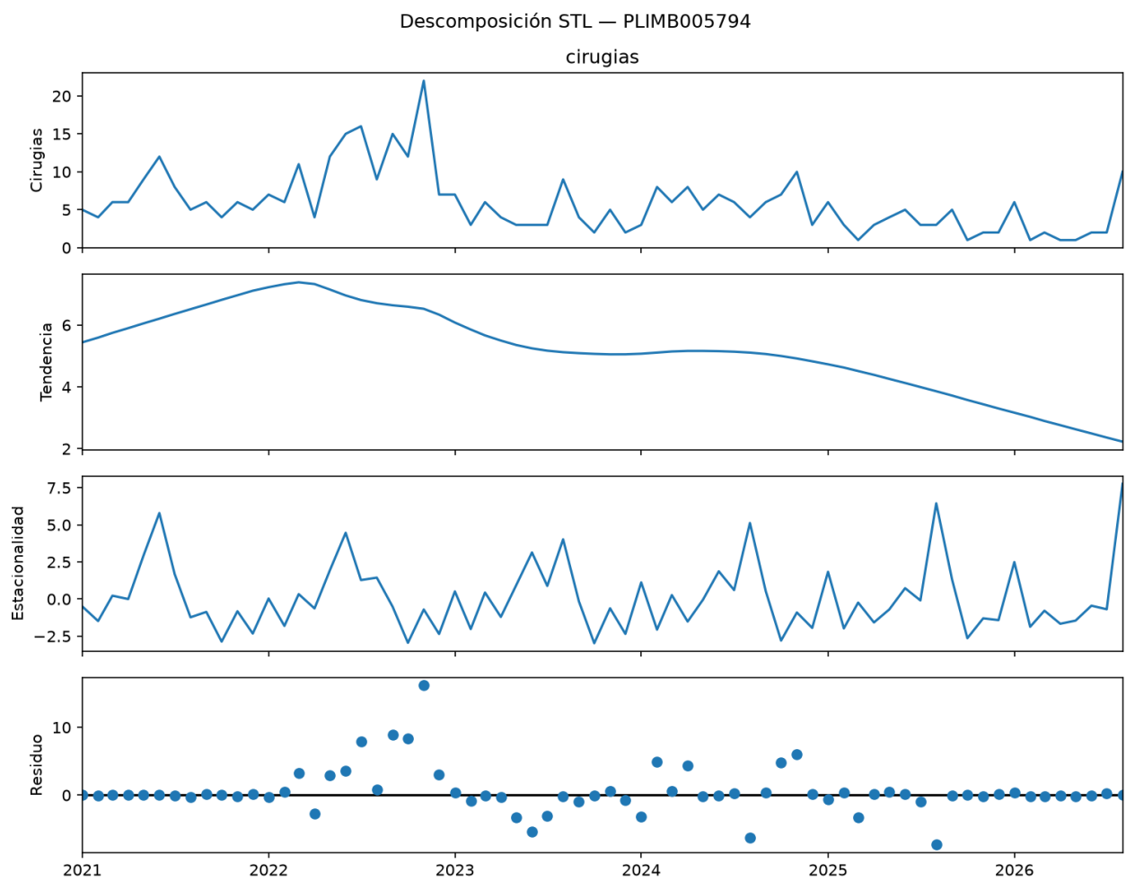
Figura 5: Descomposición STL
