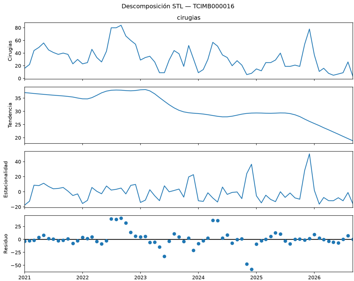
Figura 5: Descomposición STL
