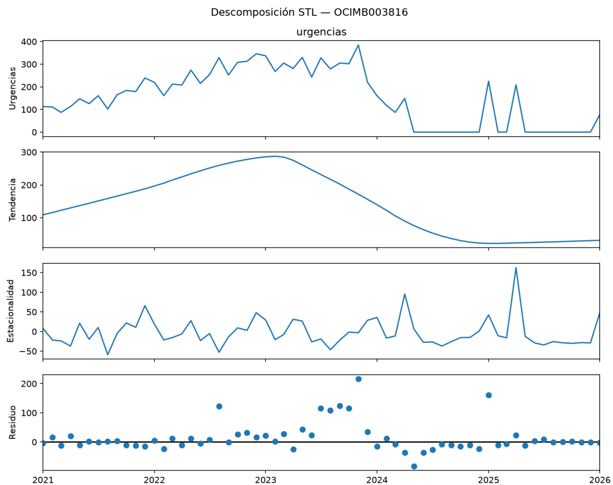
Figura 7: Descomposición STL
