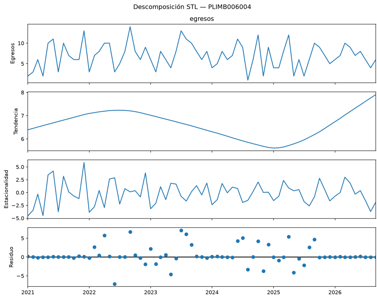
Figura 3: Descomposición STL
