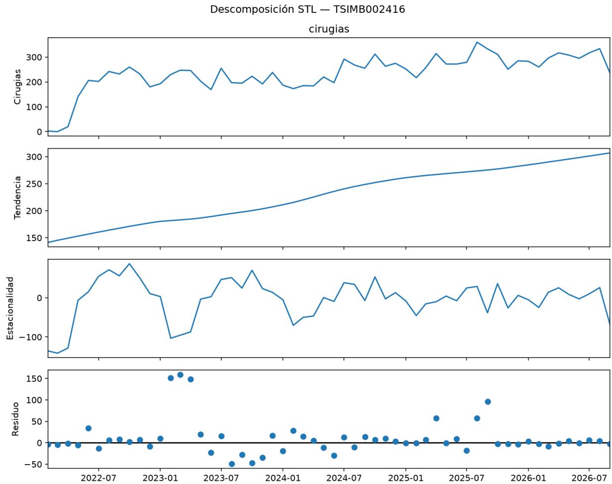
Figura 5: Descomposición STL
