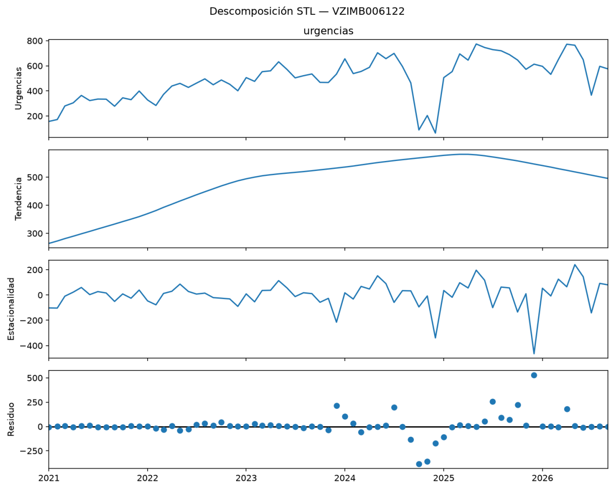
Figura 7: Descomposición STL
