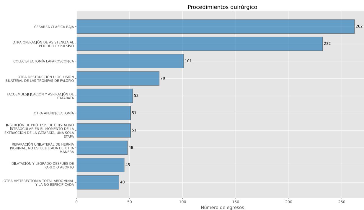
Figura 8: Procedimientos quirúrgico
