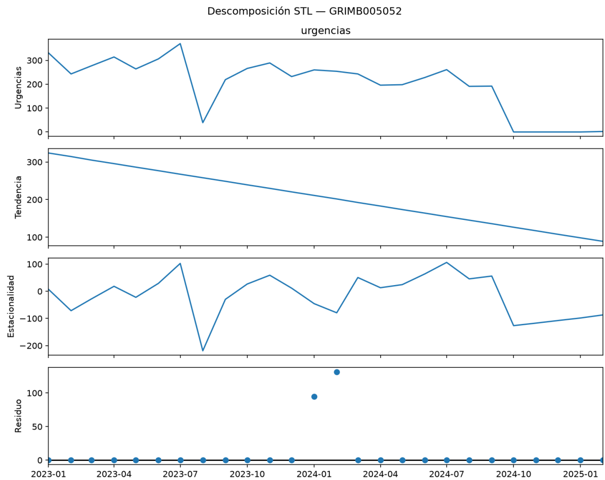
Figura 4: Descomposición STL
