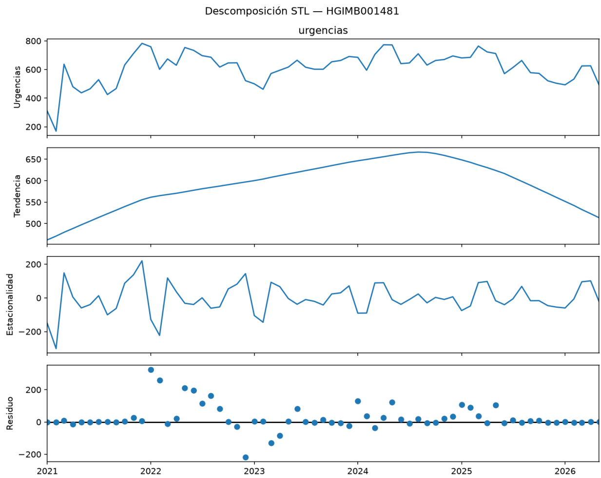
Figura 7: Descomposición STL
