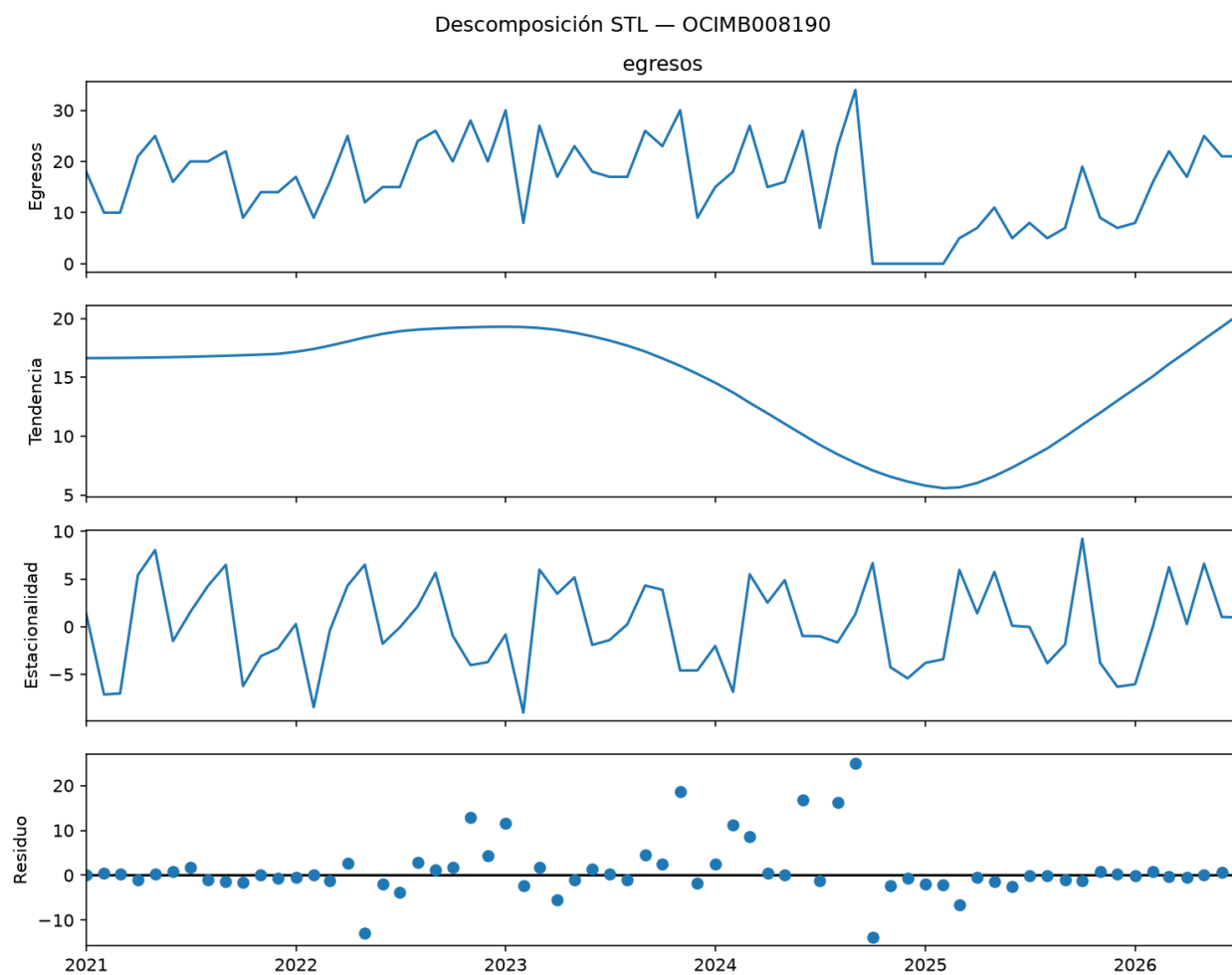
Figura 3: Descomposición STL
