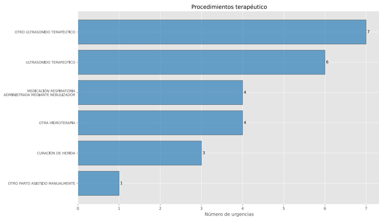
Figura 16: Procedimiento terapéutico
