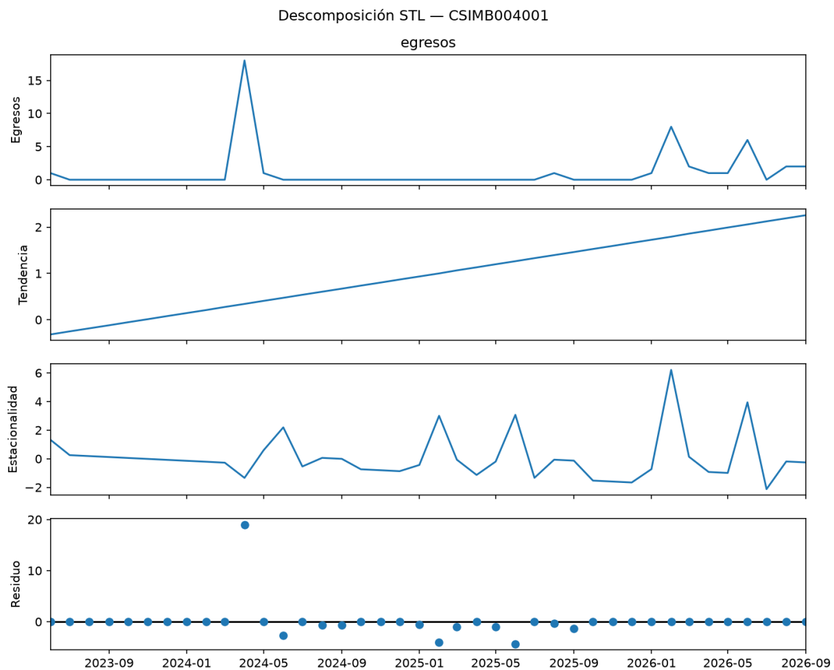
Figura 3: Descomposición STL
