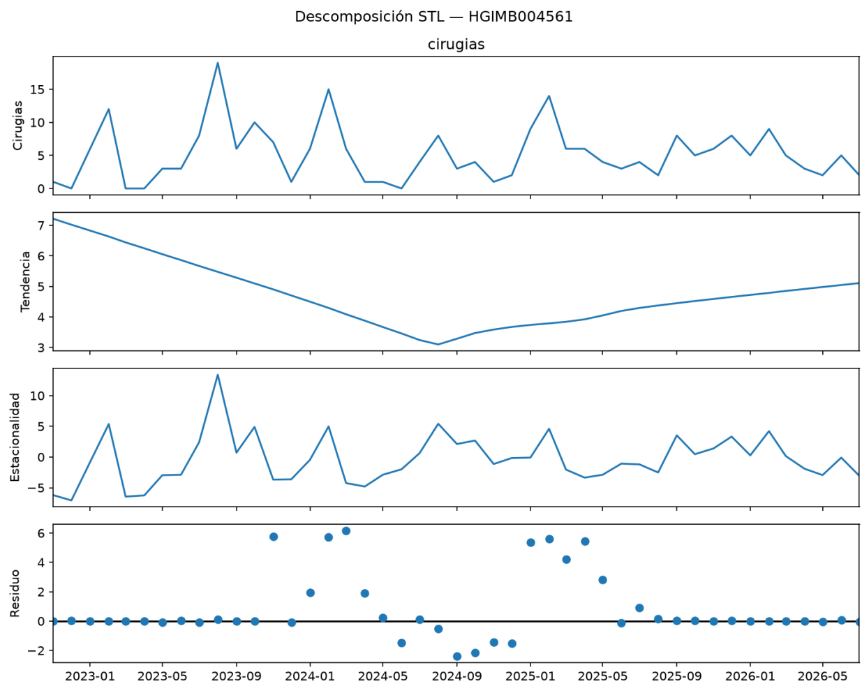
Figura 5: Descomposición STL
