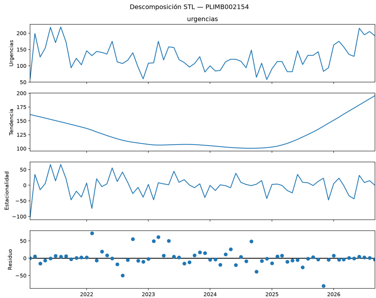
Figura 7: Descomposición STL
