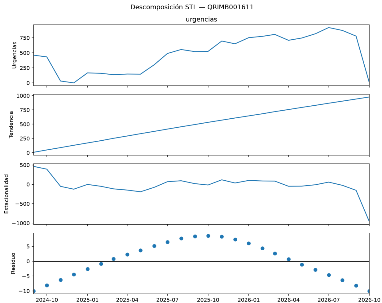
Figura 4: Descomposición STL
