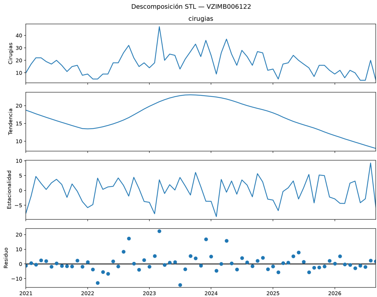
Figura 5: Descomposición STL
