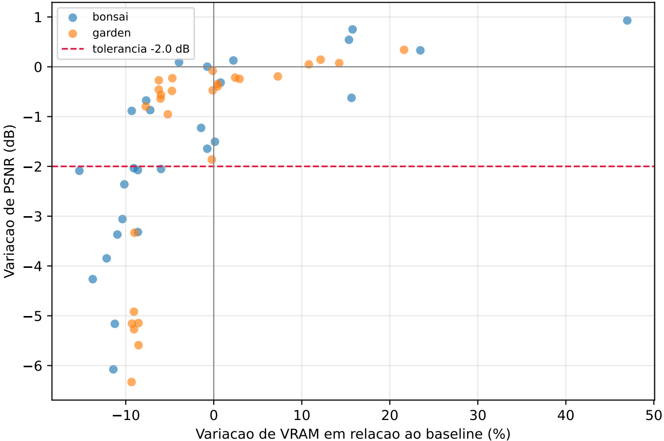
Degradacao de qualidade x economia de memoria
