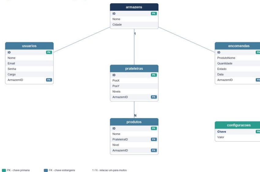
Figura 2 - Modelo de dados (diagrama entidade-rela  o).
