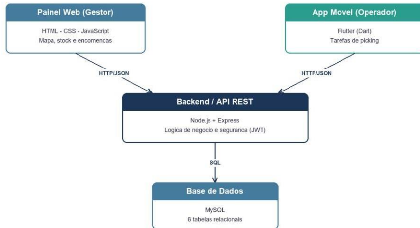
Figura 1 - Arquitetura cliente-servidor da soluç o.
