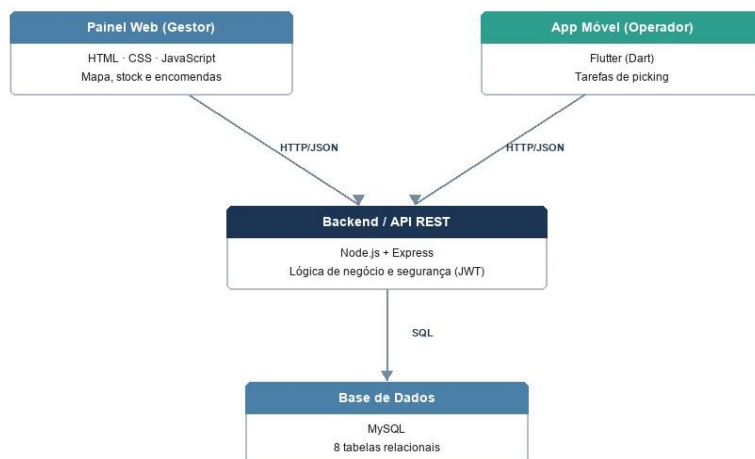
Figura 2 - Arquitetura cliente-servidor da solução.
