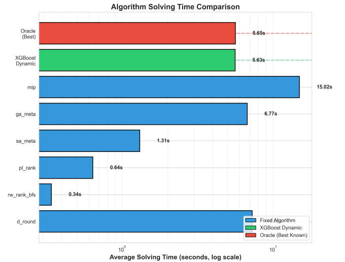
Fig. 4. Comparação de Tempo de Resolução entre Algoritmos
