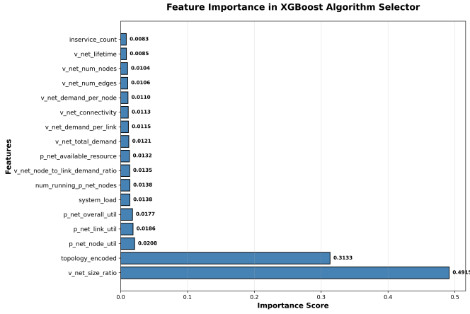
Fig. 2. Importância das Features no Modelo XGBoost
