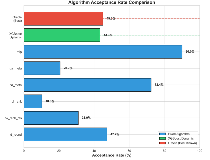
Fig. 3. Comparação de Taxa de Aceitação entre Algoritmos
