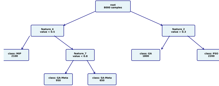
Árvore de Decisão Treinada para Seleção de Algoritmo VNE
