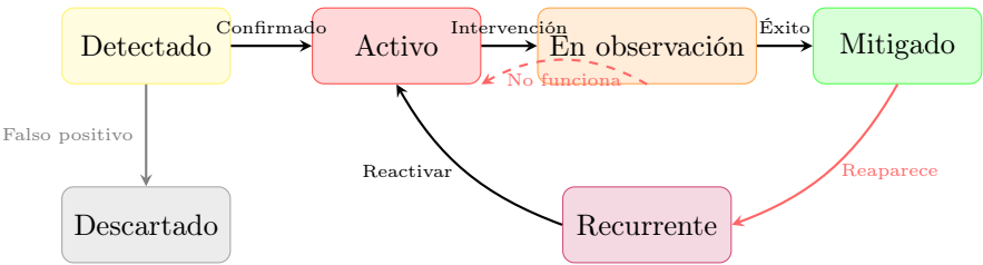
Figura 4.13: Diagrama de transición de estados de community smells
