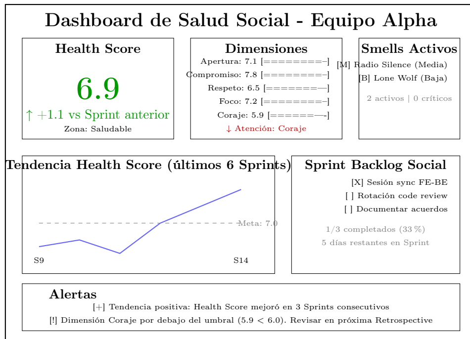
Figura 4.14: Ejemplo de Dashboard de Métricas Sociales
