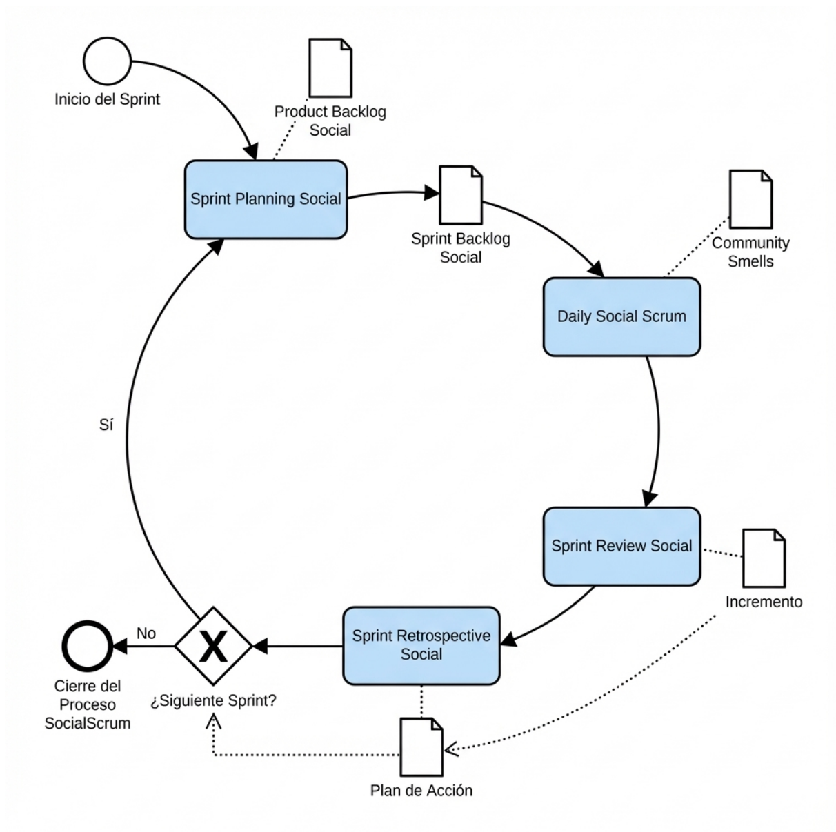
Figura 3.2: Diagrama general del proceso SocialScrum.
