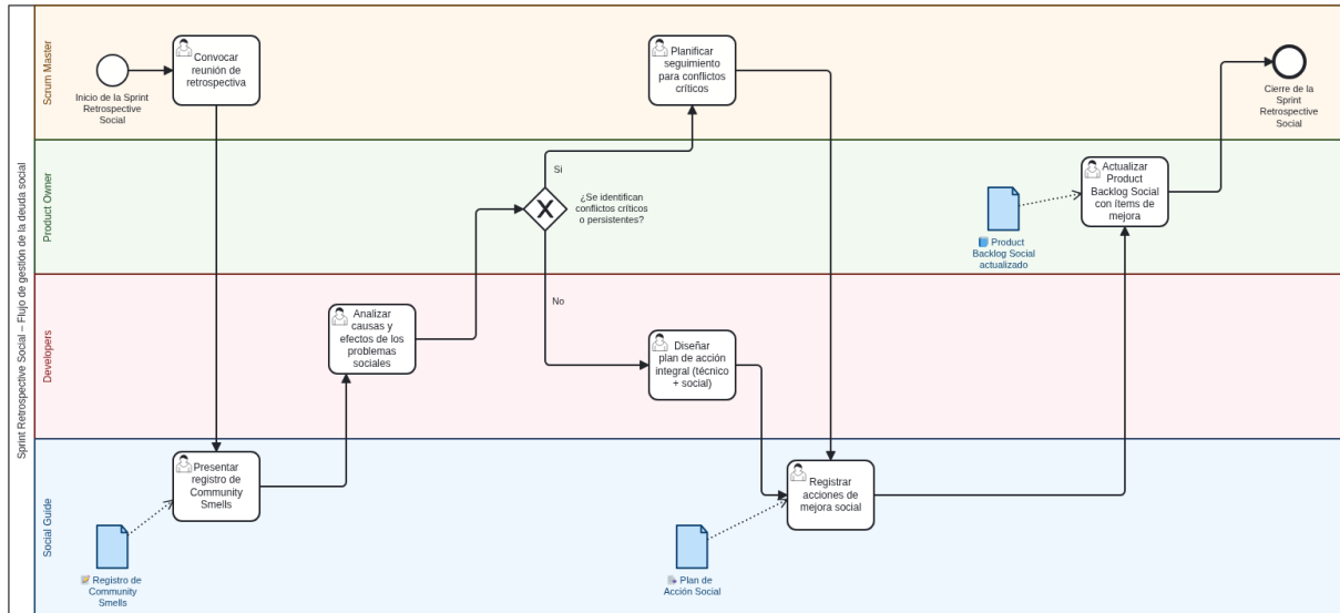
Figura 3.4: Flujo detallado del evento Sprint Retrospective Social en el modelo SocialScrum.
