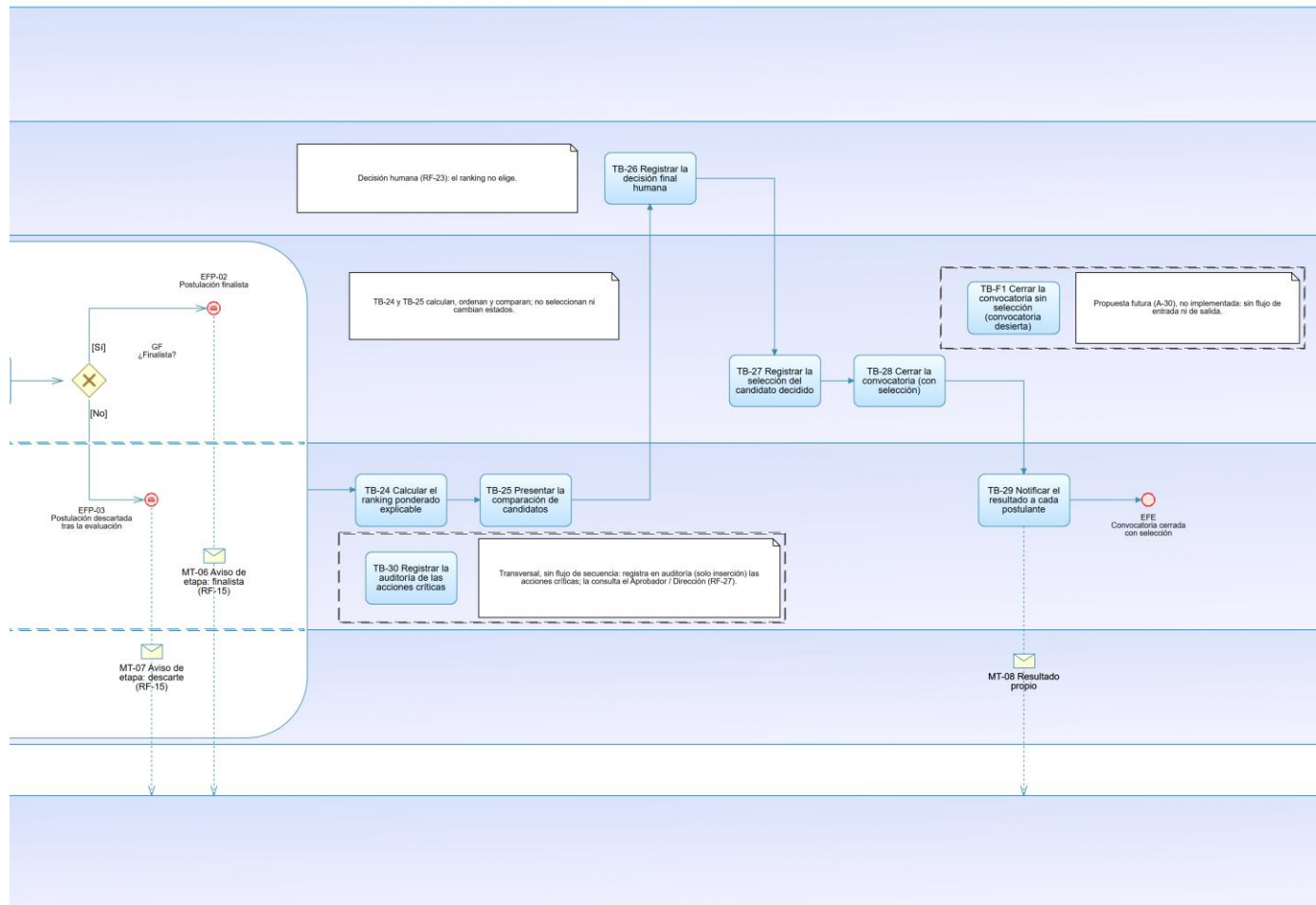
Figura 5. Ampliación de la figura 1 (franja del 72 % al 100 % del ancho): fin de SP-P y nivel vacante: ranking, decisión humana, selección y cierre (TB-24 a TB-29, EFE), TB-30 y TB-F1. Recorte sin retoque de la exportación formal.
