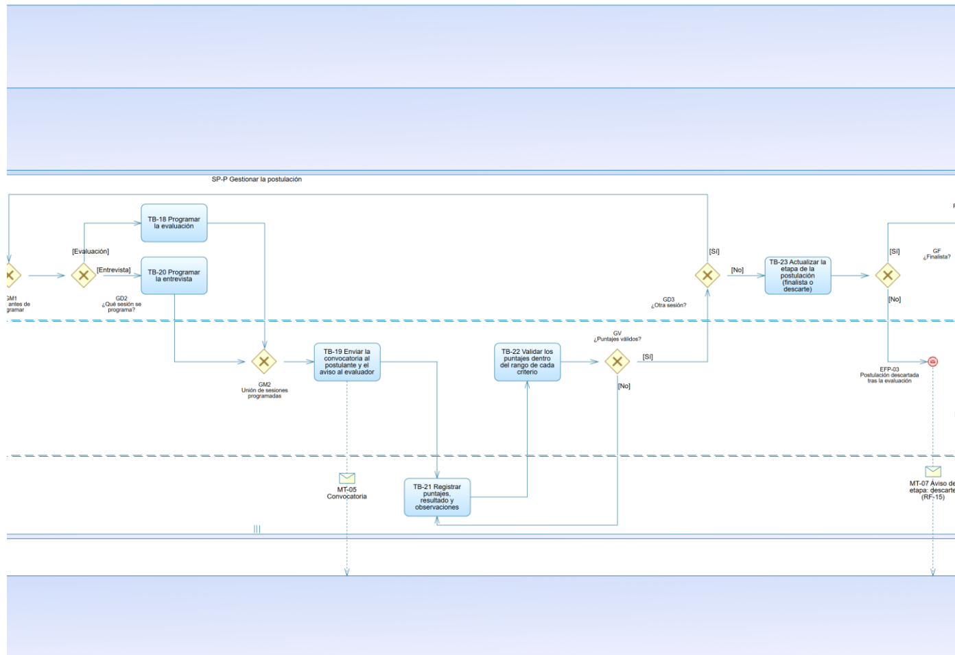
Figura 4. Ampliación de la figura 1 (franja del 48 % al 76 % del ancho): SP-P, continuación: sesiones, evaluación y entrevista (TB-18 a TB-23). Recorte sin retoque de la exportación formal.
