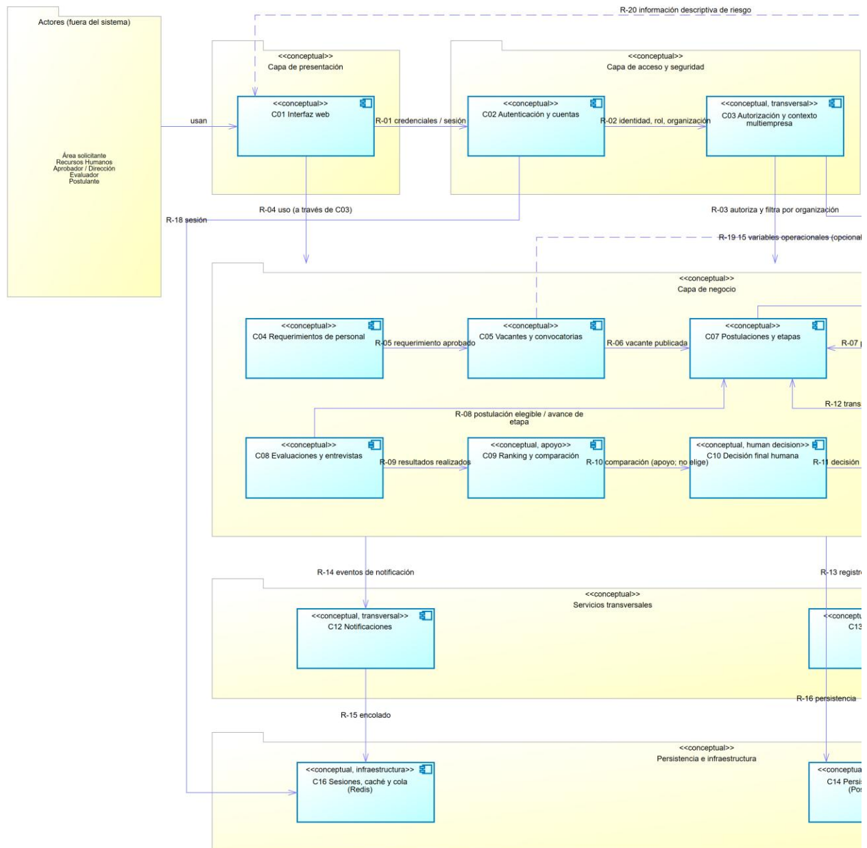
Figura 2. Ampliación de la figura 1 (franja del 0 % al 55 % del ancho). Recorte sin retoque de la exportación formal.
