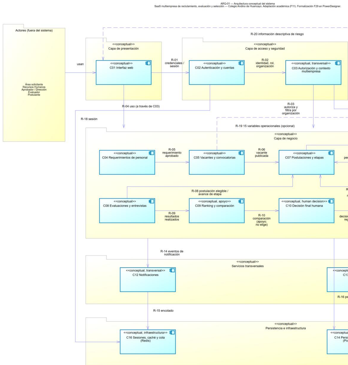
Figura 2. Ampliación de la figura 1 (franja del 0 % al 55 % del ancho). Recorte sin retoque de la exportación.
