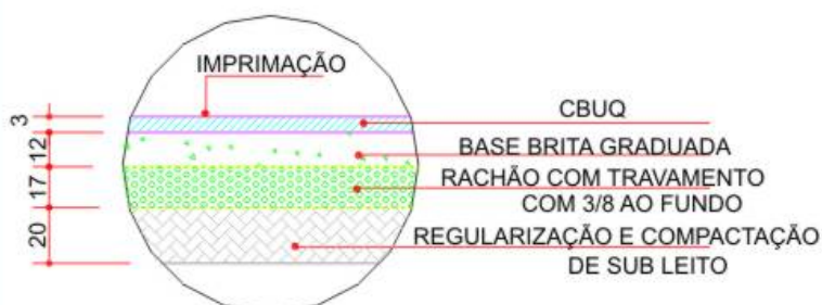
PAVIMENTAÇÃO - TRÁFEGO PESADO SEM ESCALA
