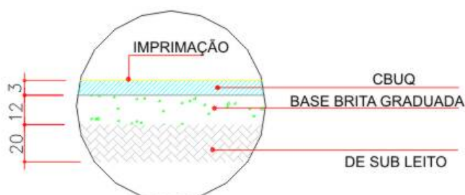
PAVIMENTAÇÃO - TRÁFEGO MÉDIO SEM ESCALA
