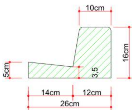
MEIO FIO TRÁFEGO LEVE, MÉDIO E PESADO SEM ESCALA
