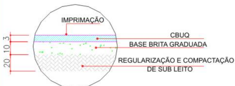
PAVIMENTAÇÃO - TRÁFEGO LEVE SEM ESCALA
