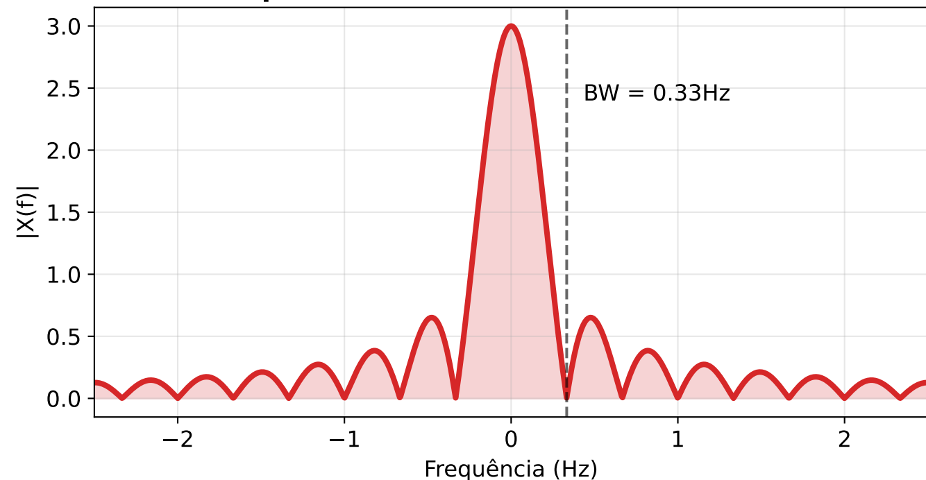
Espectro: 8-PAM (1º Nulo em 0.33 Hz)
