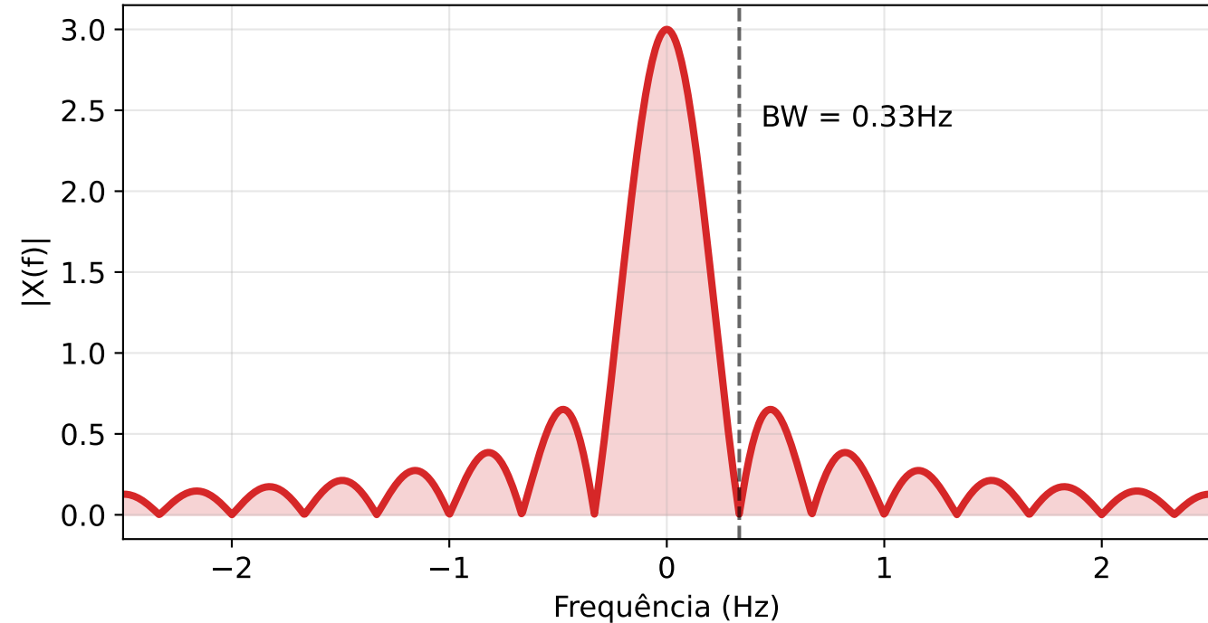
Espectro: 8-PAM (1º Nulo em 0.33 Hz)
