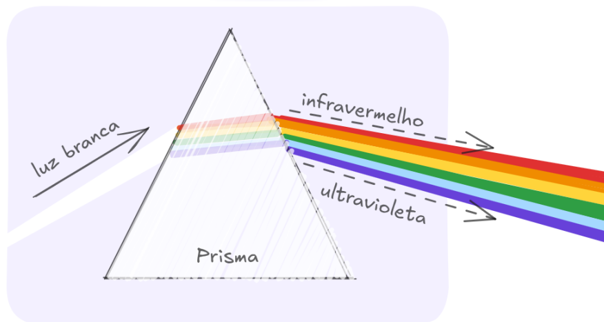
Figura 6.1: Dispersão da luz branca
