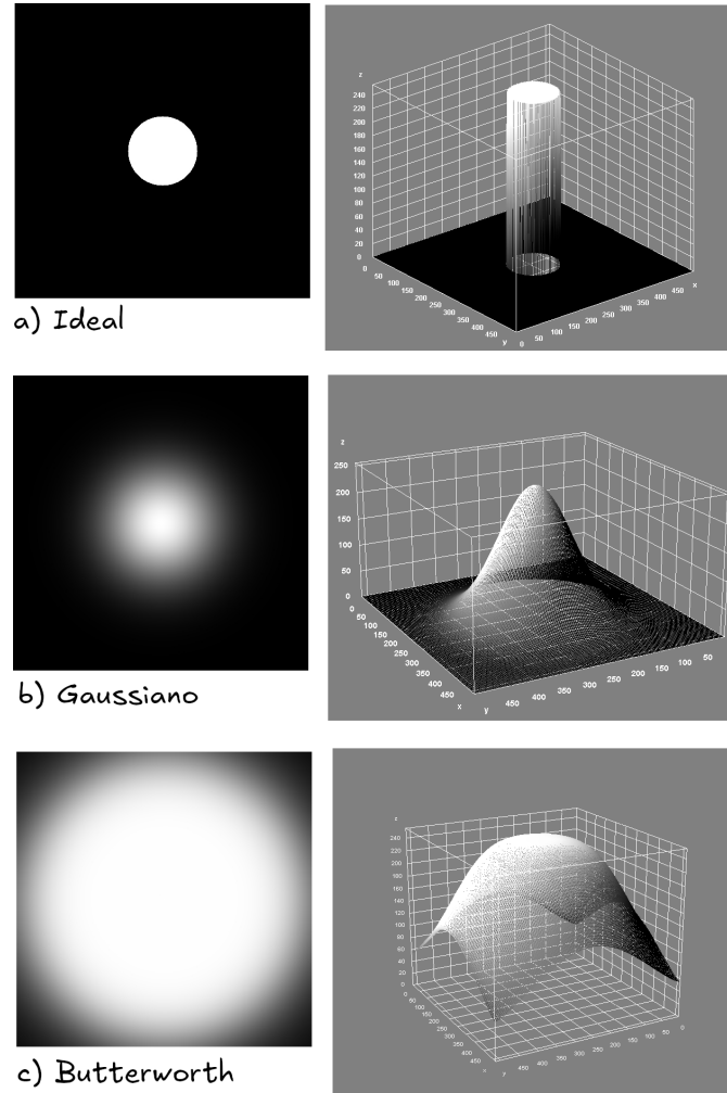
Figura 4.5: Filtros para Transformada de Fourier
