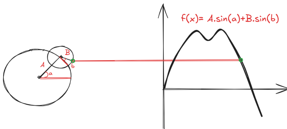
Figura 4.2: Representação dos termos como Epíclis
