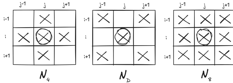
Figura 3.1: Ilustração das relações de vizinhaça dos pixels
