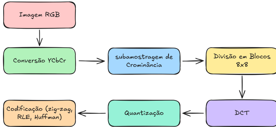
Figura 5.4: Etapas da codificação JPEG
