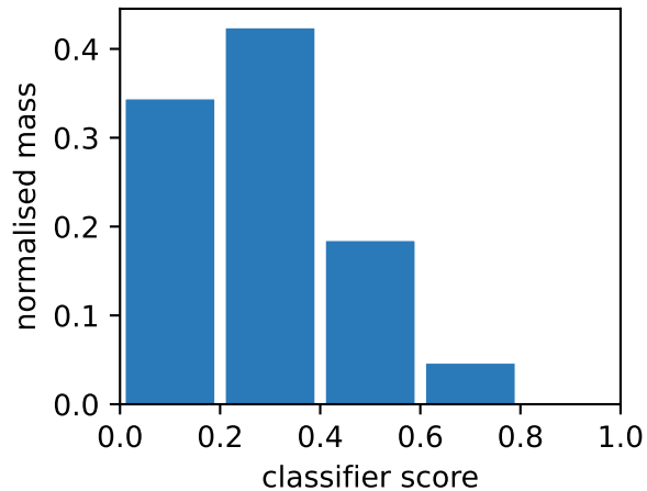
bins = 5
