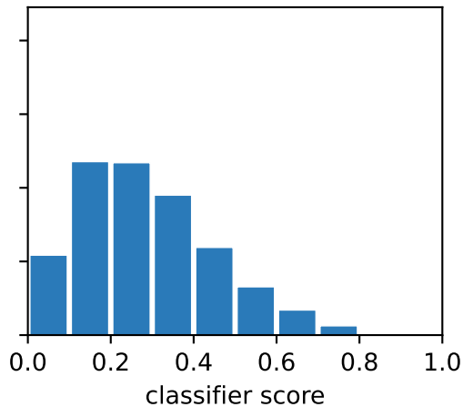
bins = 10
