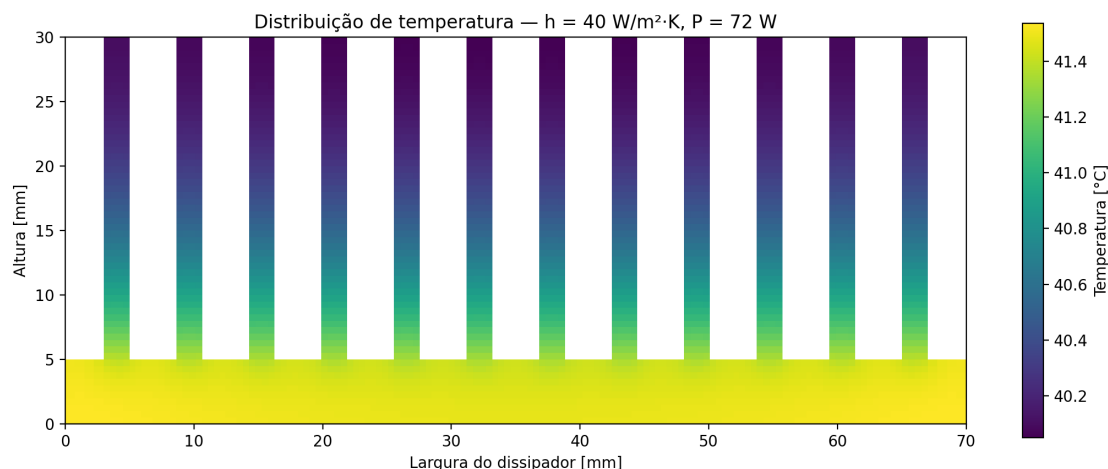
Figura 3 - Distribuição de temperatura para ventilação forçada, h = 40 \text{ W/m}^2\cdot\text{K} .
