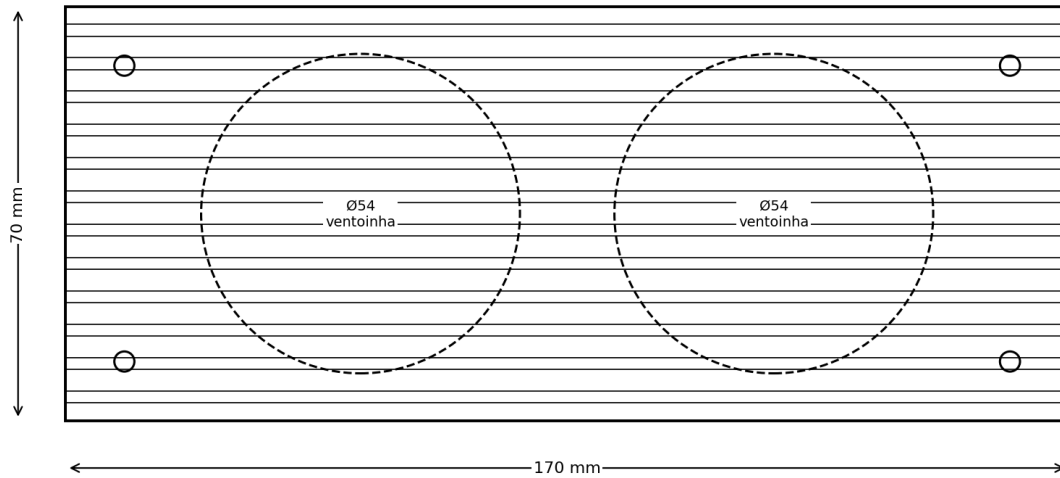
Figura B.1 - Esquema da geometria CAD integrada: dissipador, fixação conceitual e posição das ventoinhas.
