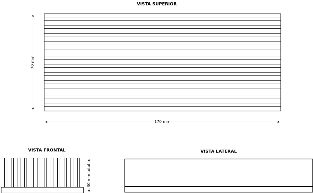
Figura 1 - Desenho técnico esquemático do dissipador proposto.
