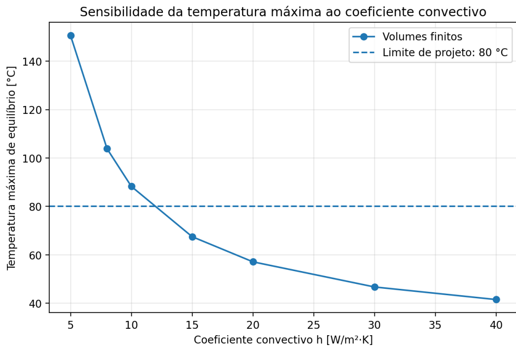
Figura 2 - Sensibilidade da temperatura máxima ao coeficiente convectivo.
