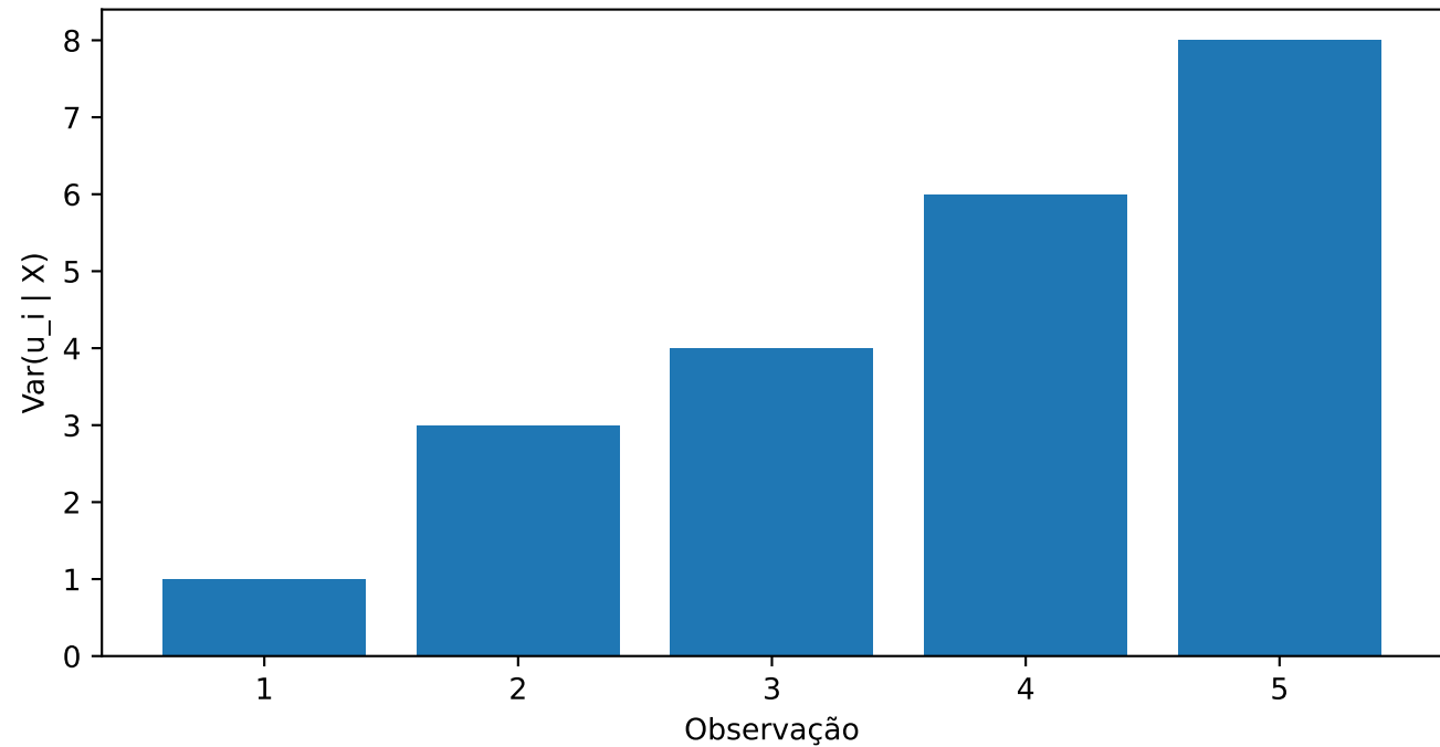
Lista 5 - Questão 5: variância condicional do erro
