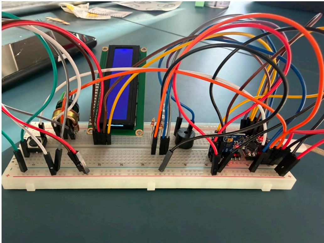
Figura 1 – Protótipo do SMN-Q montado em protoboard.
