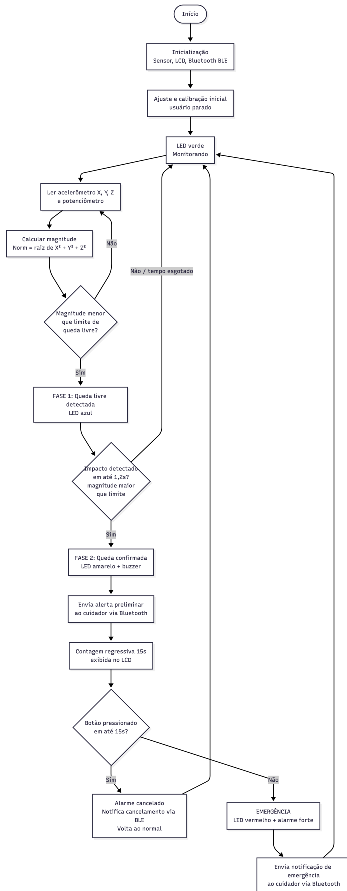
Figura 2 – Fluxograma do funcionamento do sistema SMN-Q.
