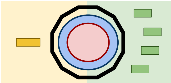
Rest API
