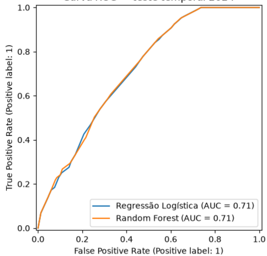
Curva ROC — teste temporal 2024
