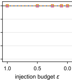
dense
