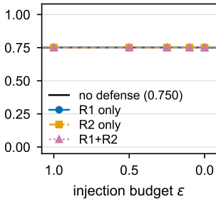
BM25
