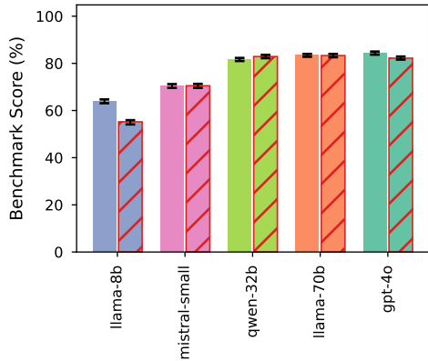
MMLU
