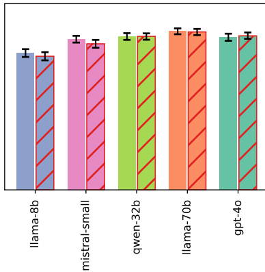
GSM8K
