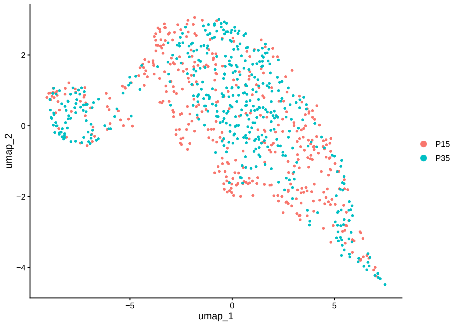
Reclustered cones: age
