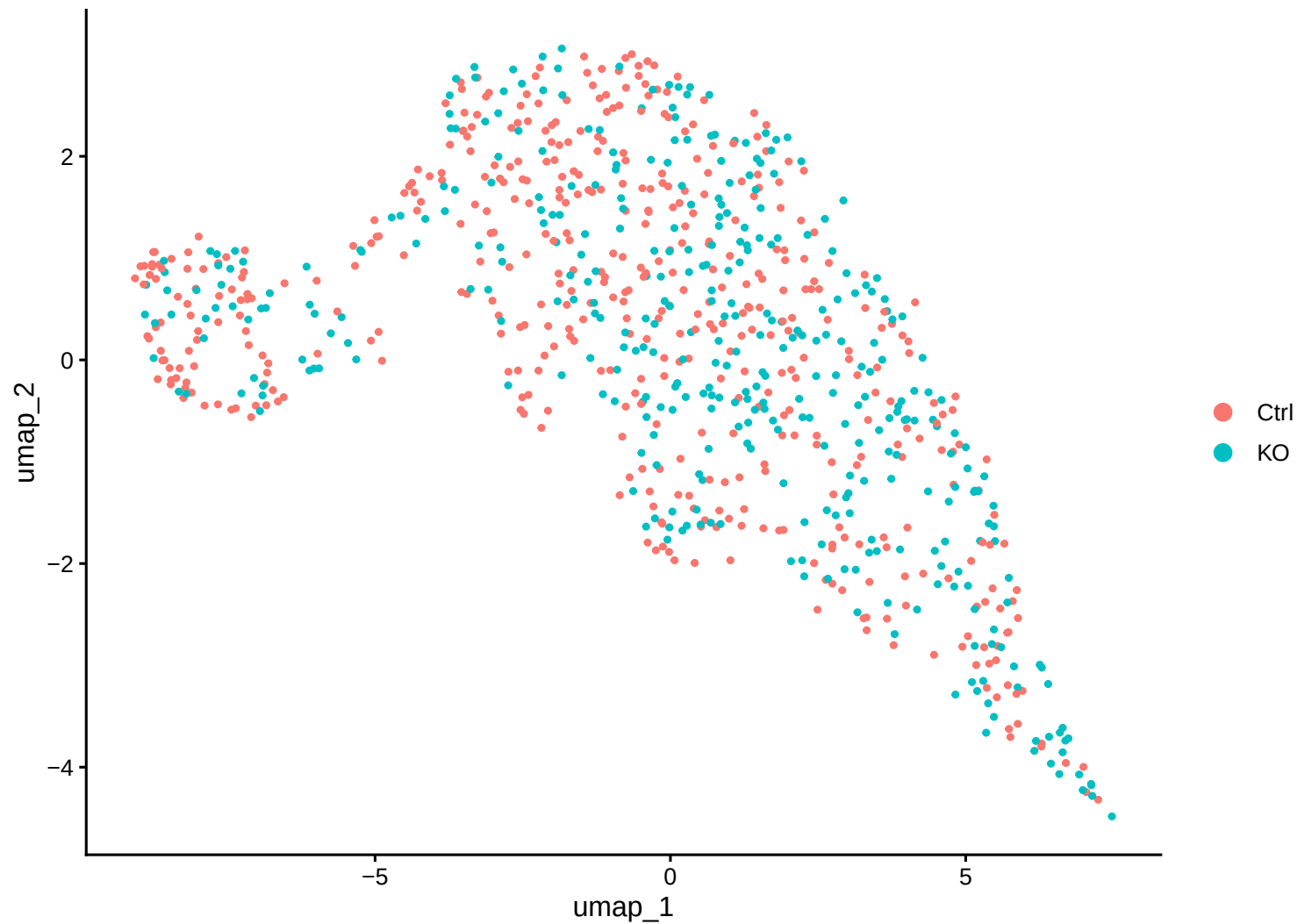
Reclustered cones: Ctrl vs KO
