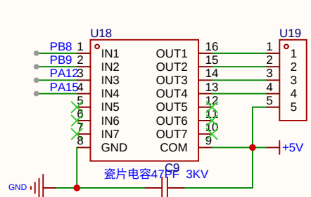
步进电机驱动
