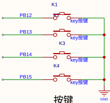
STM32F103C8T6最小系统板
