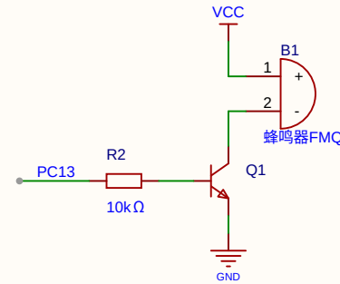
蜂鸣器
