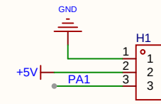
水位传感器
