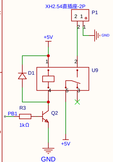
继电器
