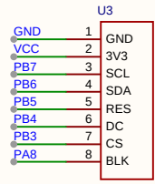
TFTLCD
