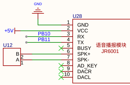
JR6001语音模块
