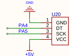
HX711称重模块
