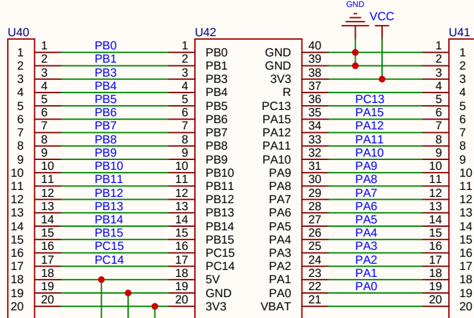
STM32F103C8T6最小系统板
