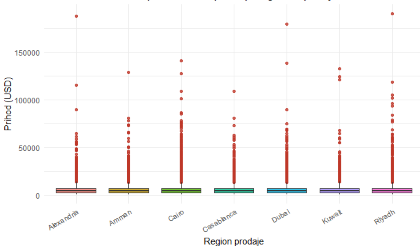
Boxplot: Ostvareni prihod po regionima prodaje
