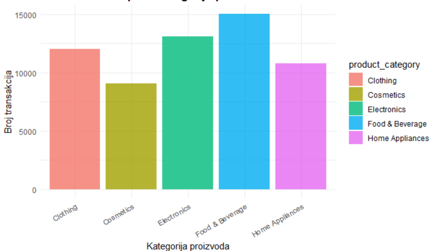
Bar plot: Kategorije proizvoda
