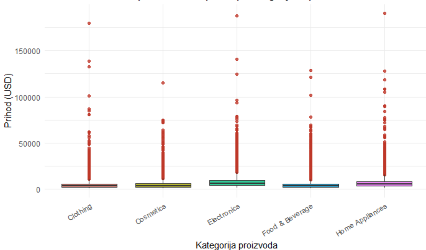
Boxplot: Ostvareni prihod po kategorijama proizvoda
