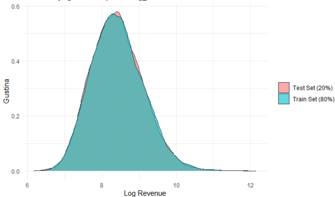
Poređenje gustine raspodele log_revenue između Train i Test seta
