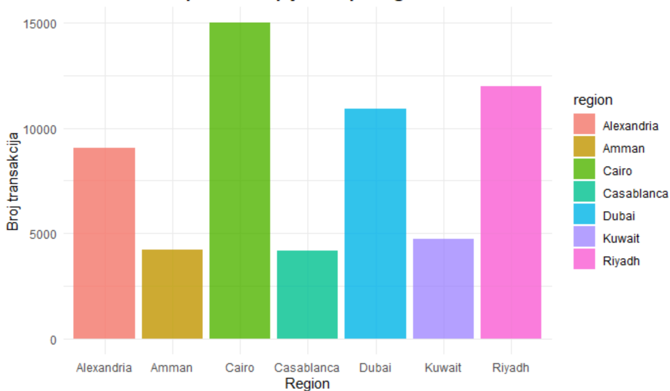
Bar plot: Zastupljenost po regionima
