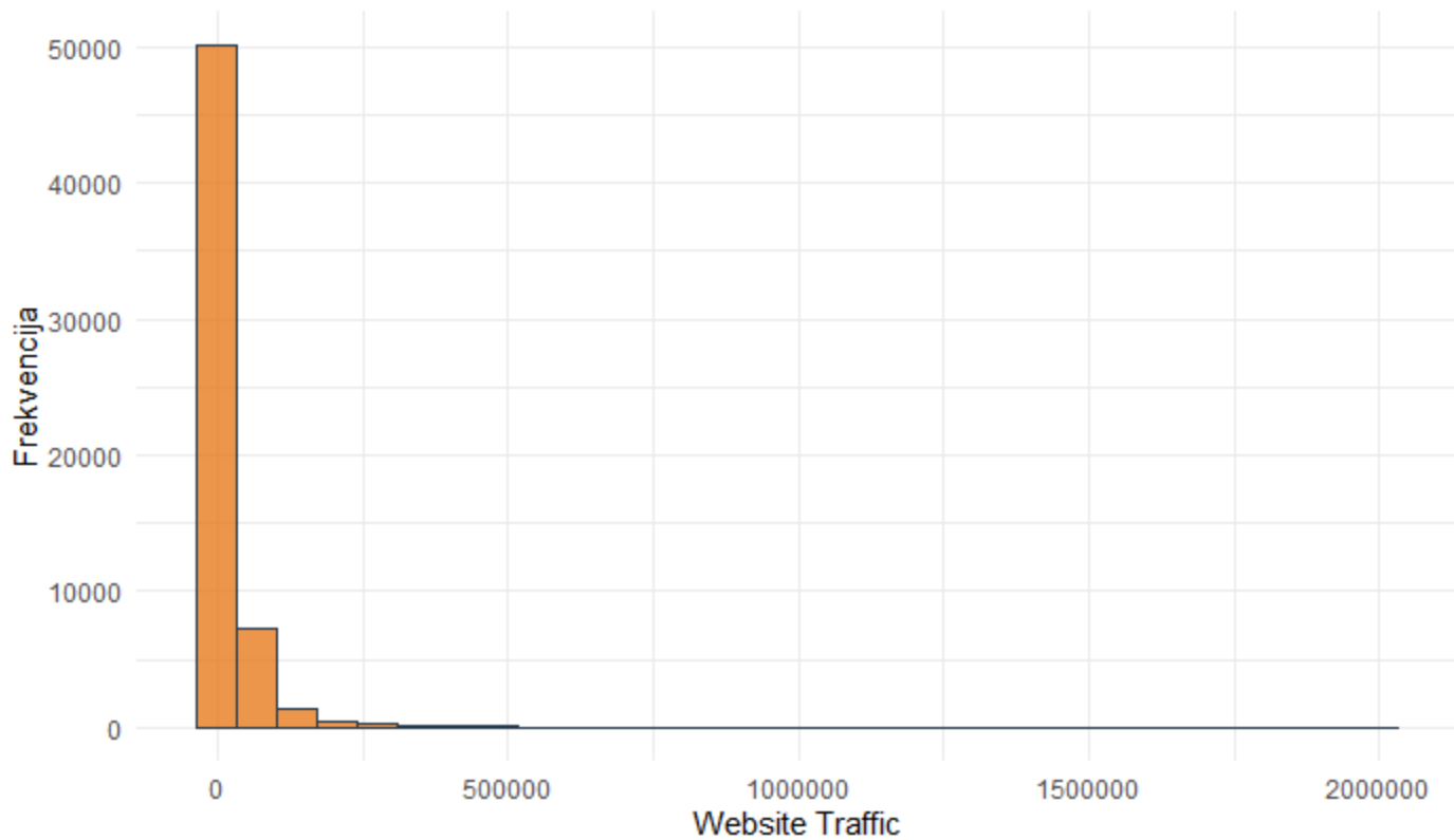
Histogram: Posete sajtu
