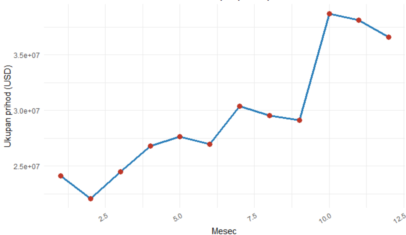
Sezonski obrasci: Ukupan prihod po mesecima
