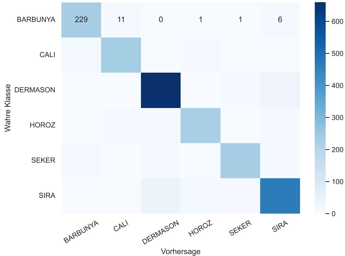
Konfusionsmatrix: MLP Neural Network
