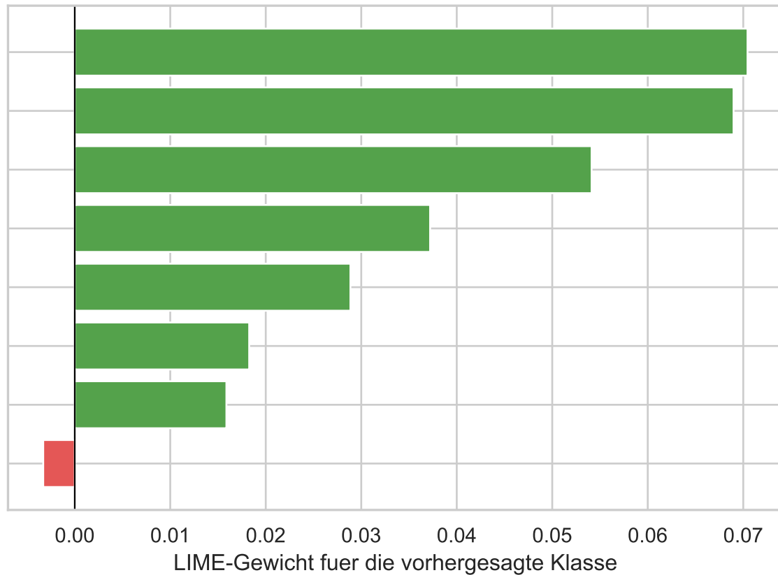
Lokale LIME-Fehlklassifikation: DERMASON als SIRA
