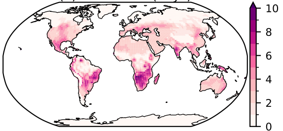
(h) SU StdDev (days)
