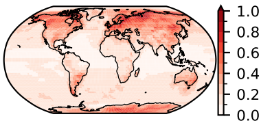
E3SMv2 (21)
