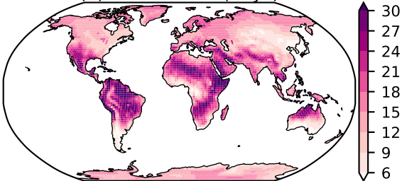
(g) SU mean (days)
