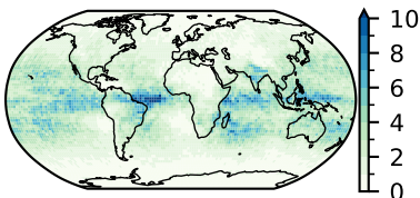
MIROC-ES2L (30)
