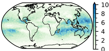
CESM2_smbb (50)
