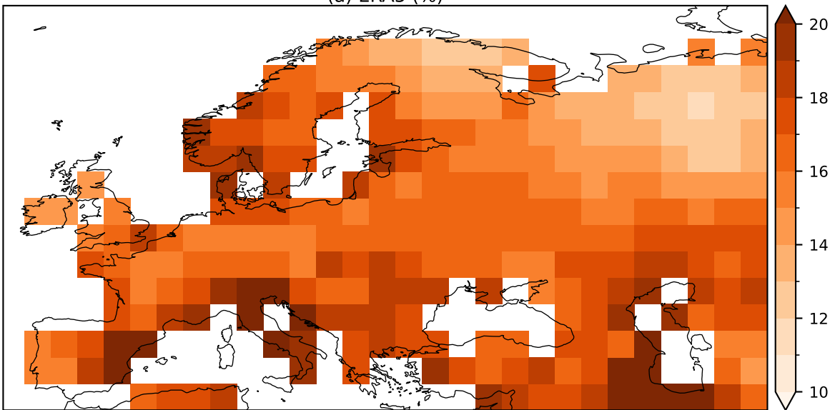
(a) ERA5 (%)
