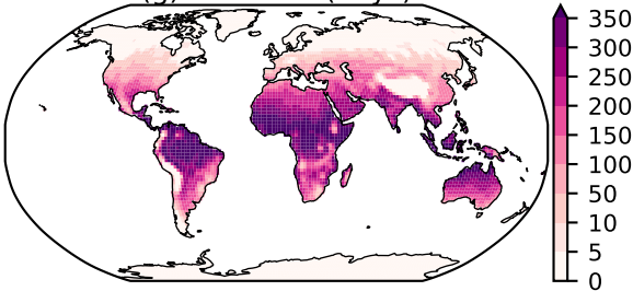
(g) SU mean (days)
