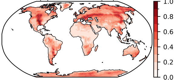
(d) TX90p StdDev (%)
