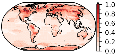
CESM2_smbb (50)
