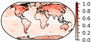
E3SM-1-0 (15)
