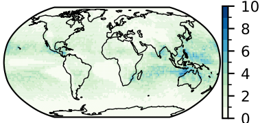
E3SMv2 (21)
