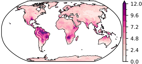
(h) SU StdDev (days)
