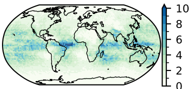
MIROC-ES2L (30)
