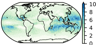
CESM2_smbb (50)
