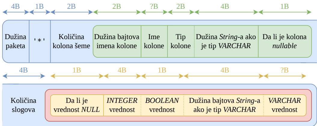
Slika 29: Struktura QuerySet paketa
