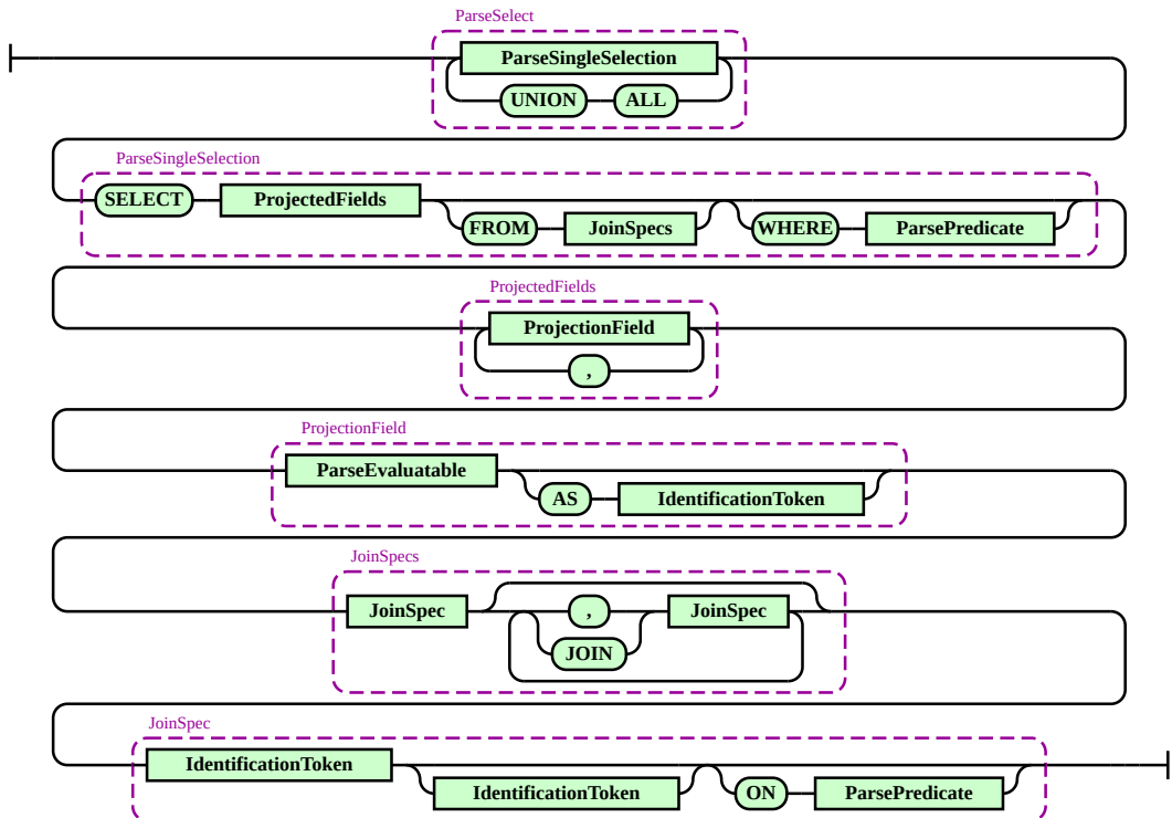
Slika 12: Gramatika ParseSelect sintaktičke kategorije
