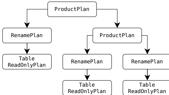
Slika 25: Primer stabla planova nakon proizvoda 3 tabele
