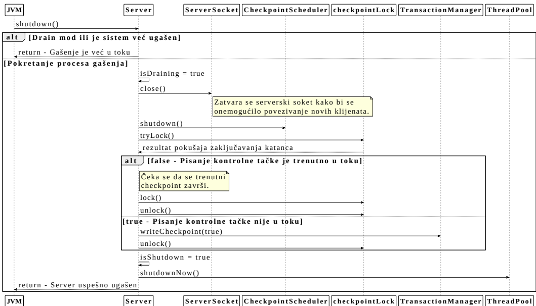
Slika 31: Dijagram sekvence bezbednog gašenja servera
