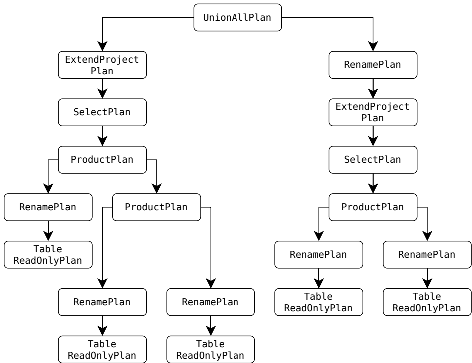
Slika 27: Primer kompletnog stabla planova
