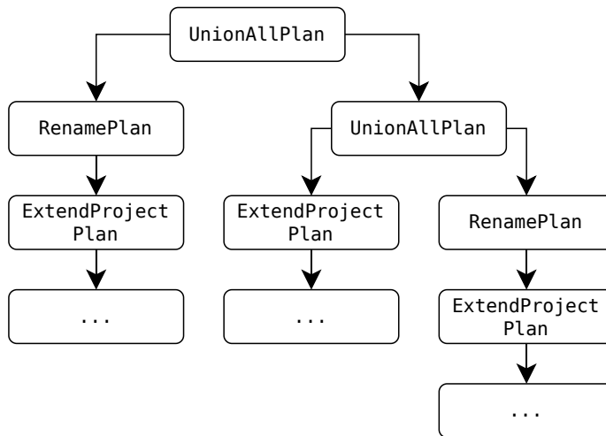
Slika 23: Primer stabla planova nakon unije 3 naredbe
