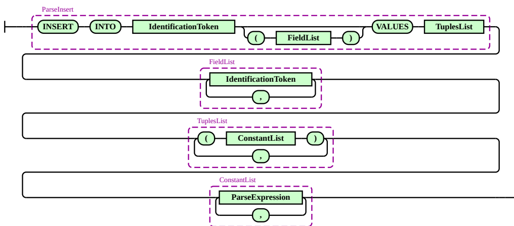
Слика 13: Gramatika ParseInsert sintaktičke kategorije
